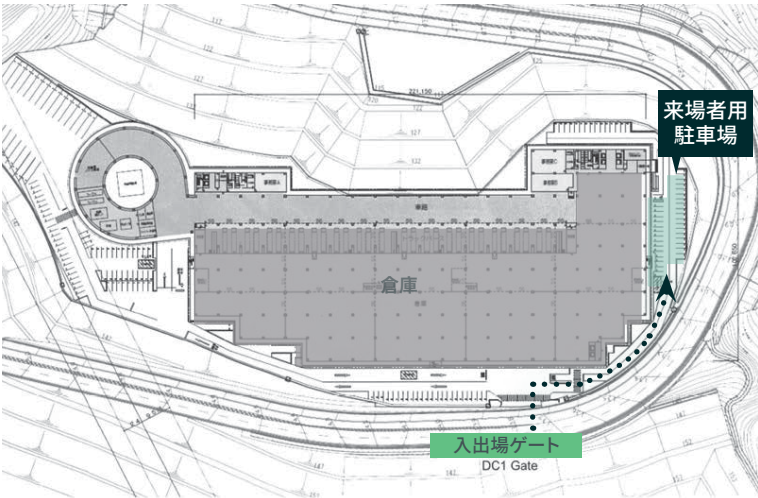
3F 平面図
