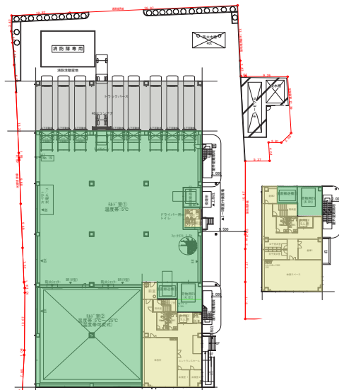
配置図・1-2F 平面図
